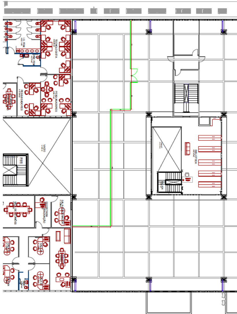
Figura 01: Planta situacional da instalação do gradil nas UTAs do Piso Técnico do ICC
